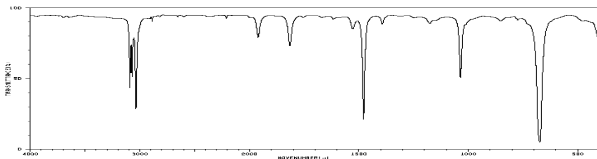
Рис. 4. ИК-спектр бензола
